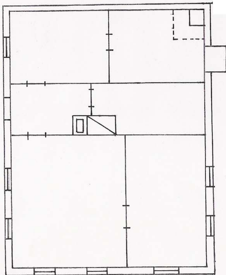
План деревянного одноэтажного дома пермского мещанина М.Ф. Малых в I части г. Перми по II мещанской улице. № 14. ГАПО. Ф. 716. Оп. 1. Д. 719.
