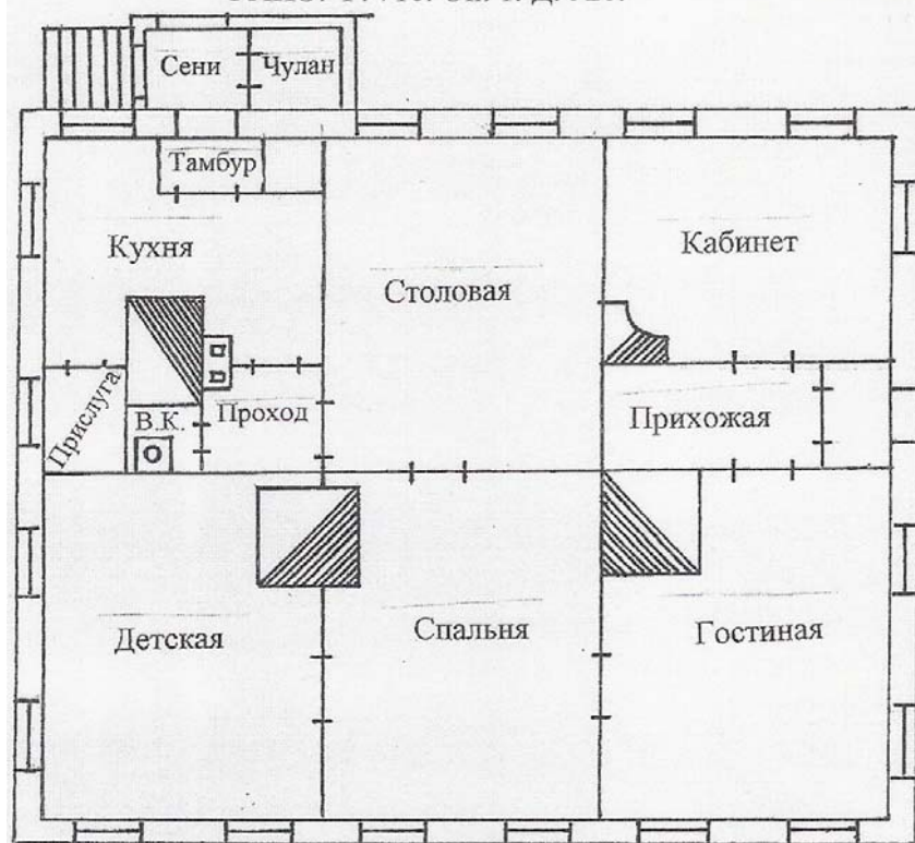
Вариант квартиры служащих завода «Электросталь» ГАПО. Ф. 716. Оп. 1. Д. 928.
